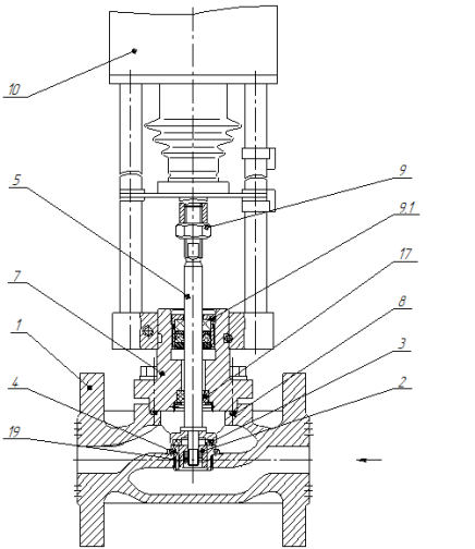
Рисунок 2. Неразгруженный по давлению клапан DN 15 – 40. Исполнение А.
