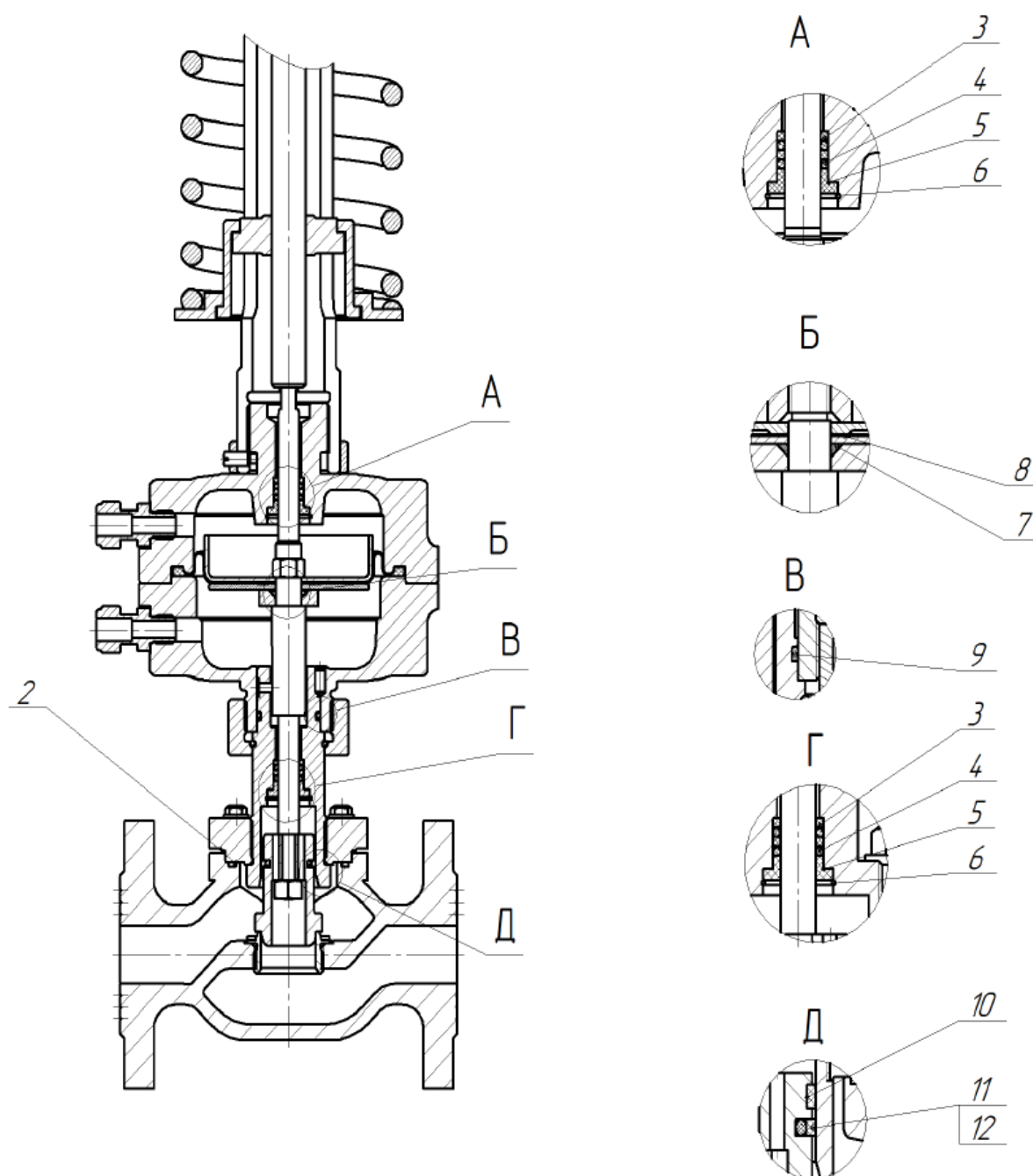
Рис. 5. Ремкомплекты
