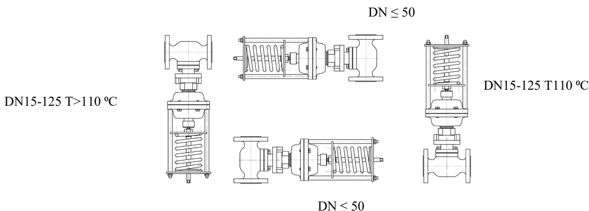
Рис. 3. Схема монтажных положений регулятора давления прямого действия РА-В
