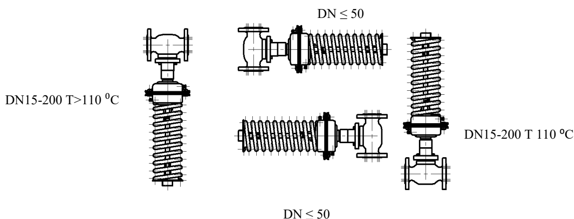
Рис. 3. Схема монтажных положений регулятора давления прямого действия РА-В
